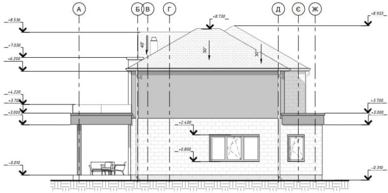
1 Фасад А-Ж 1:75
